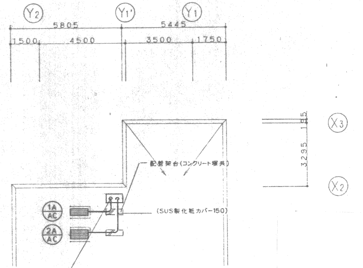
R階平面図 S=1/100
