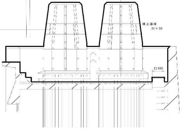
断面詳細図
