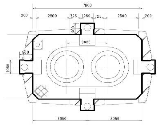
平面詳細図
