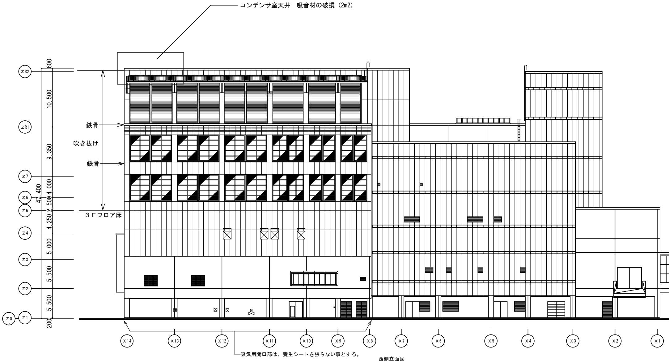
西側立面図 1/400
