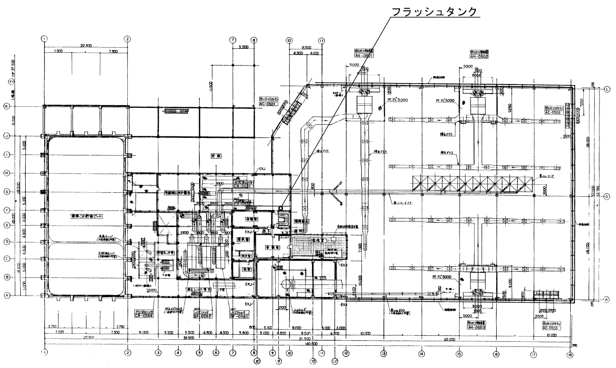
2階平面図
