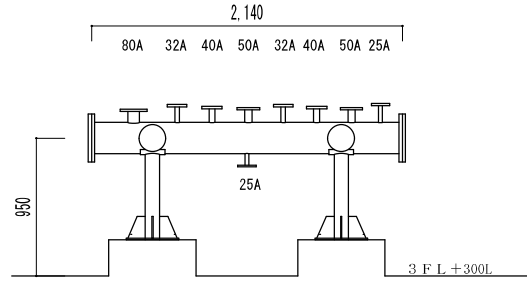
給湯用ヘッダー（リターン側）
