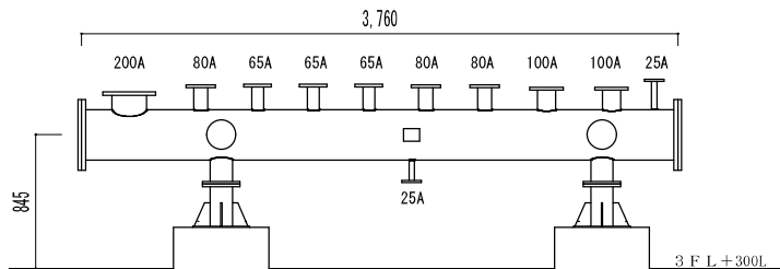
暖房用ヘッダー（リターン側）
