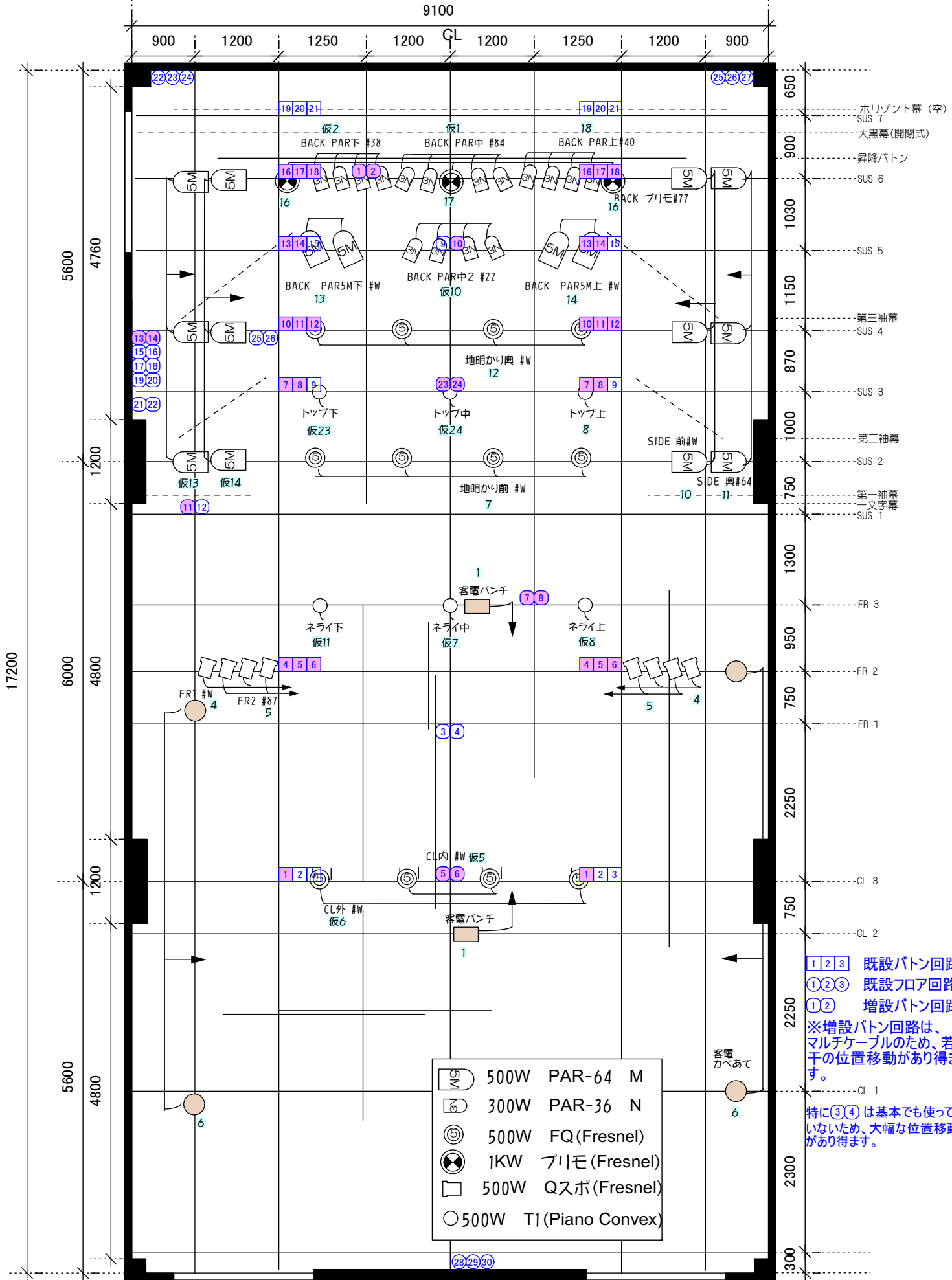
照明基本仕込み図 ※番号は使用回路。番号のみはボックス、「仮」はマルチ TITLE 照明回路図 ※塗りつぶしは基本仕込で使用中的のもの
