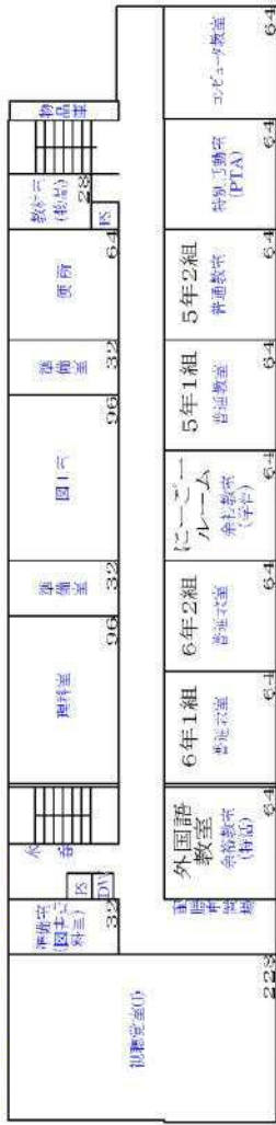
4 階平面図
