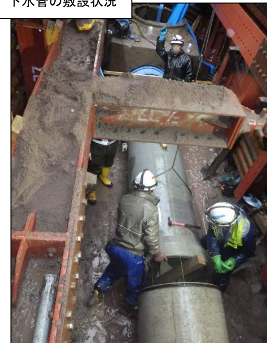
下水管の敷設状況
