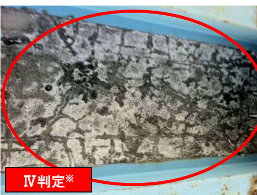
【鋼橋の床版】ひび割れ：Ⅳ判定相当
