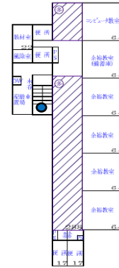
3階平面図
