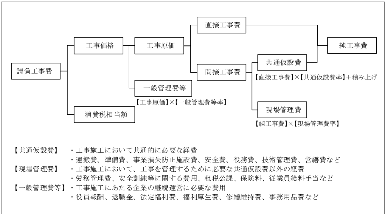
図2 工事費の構成（土木工事の場合）
