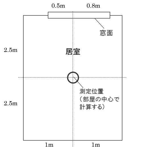
▲平面図
