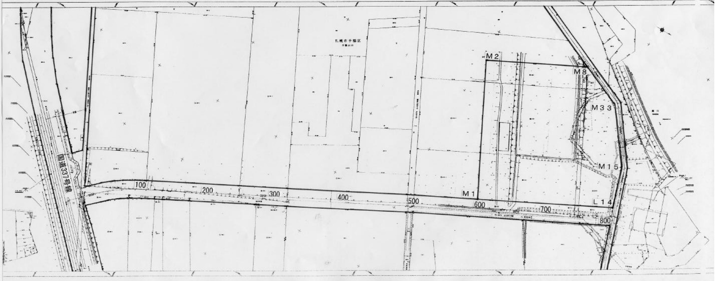
別紙-2-① 山口東2号線予備設計図-1 国道からのアプローチ路
