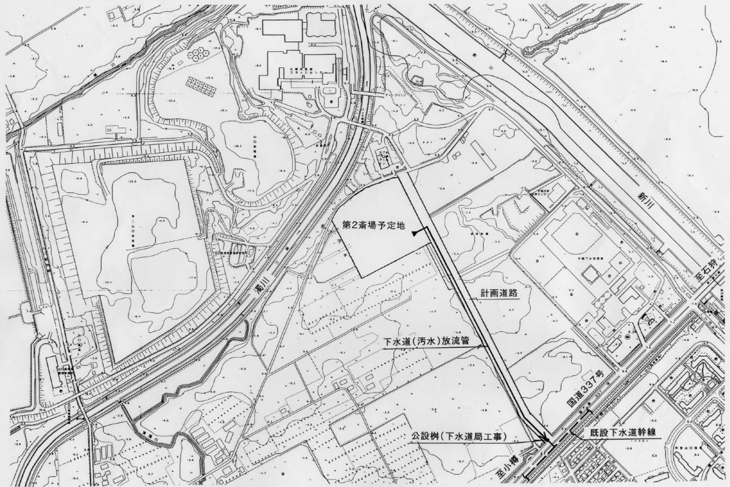
別紙-13 下水道(汚水)放流計画図(S=1/5000)
