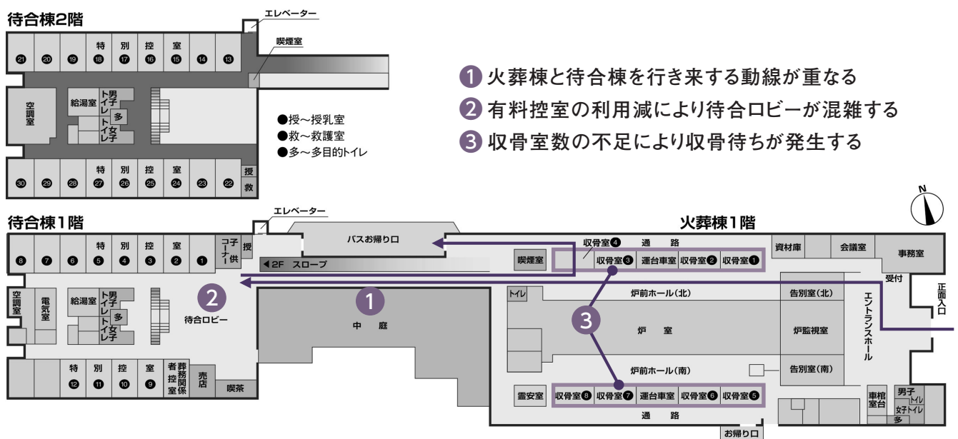
【図3-7 里塚斎場の見取図とその構造上の問題点】
