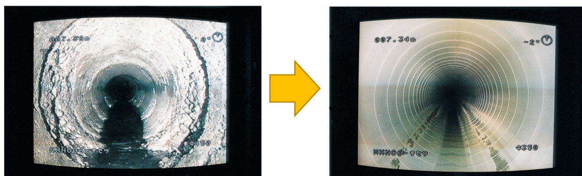
管更生工法による管路の改築
