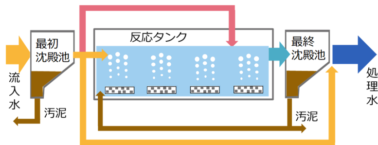
雨天時下水活性汚泥法
