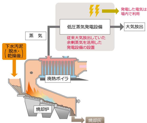
蒸気発電（汚泥処理の過程で発生する蒸気を活用して発電）
