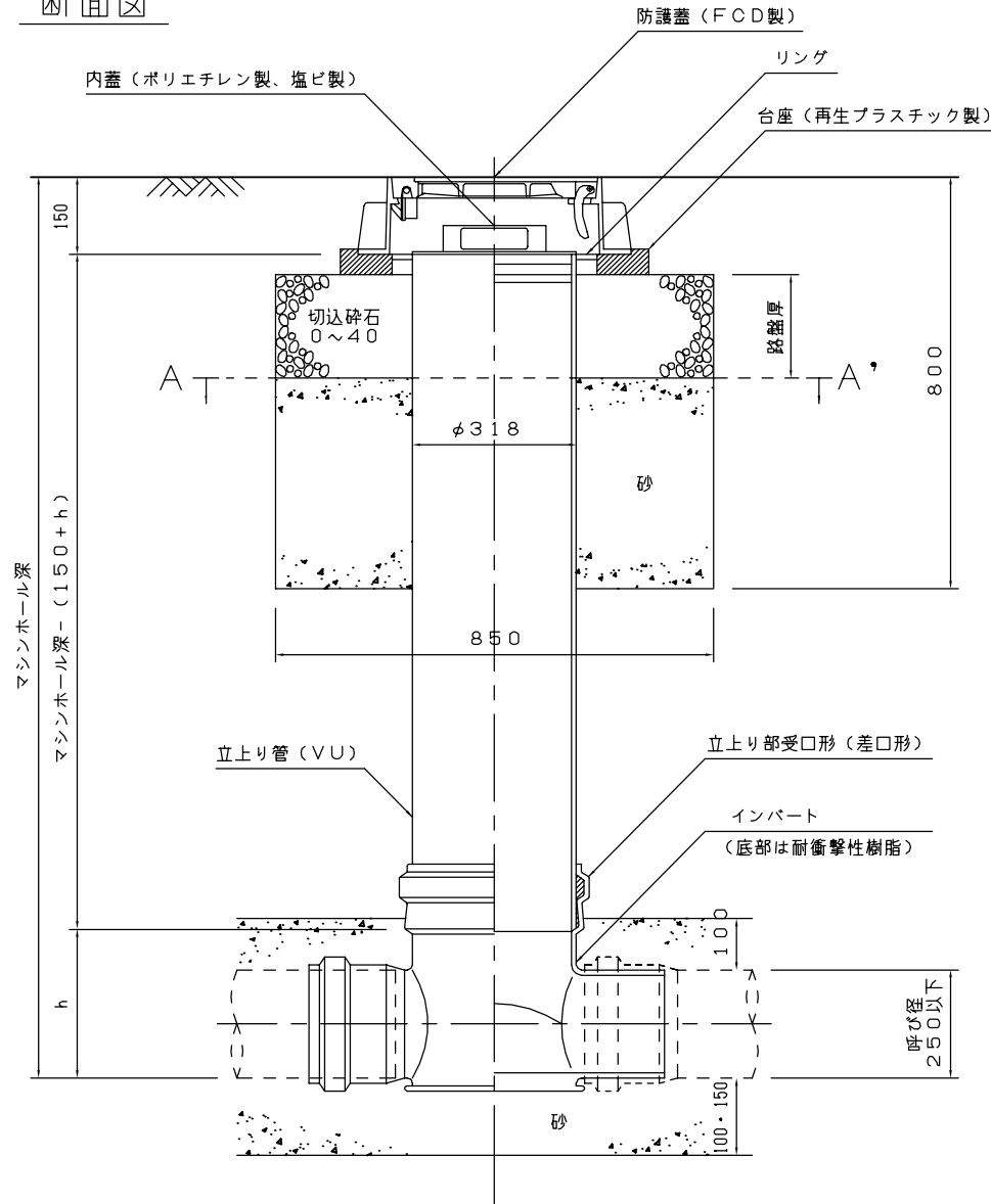
断面図
