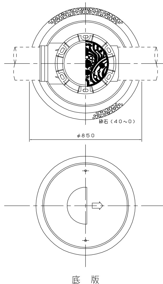
平面図
