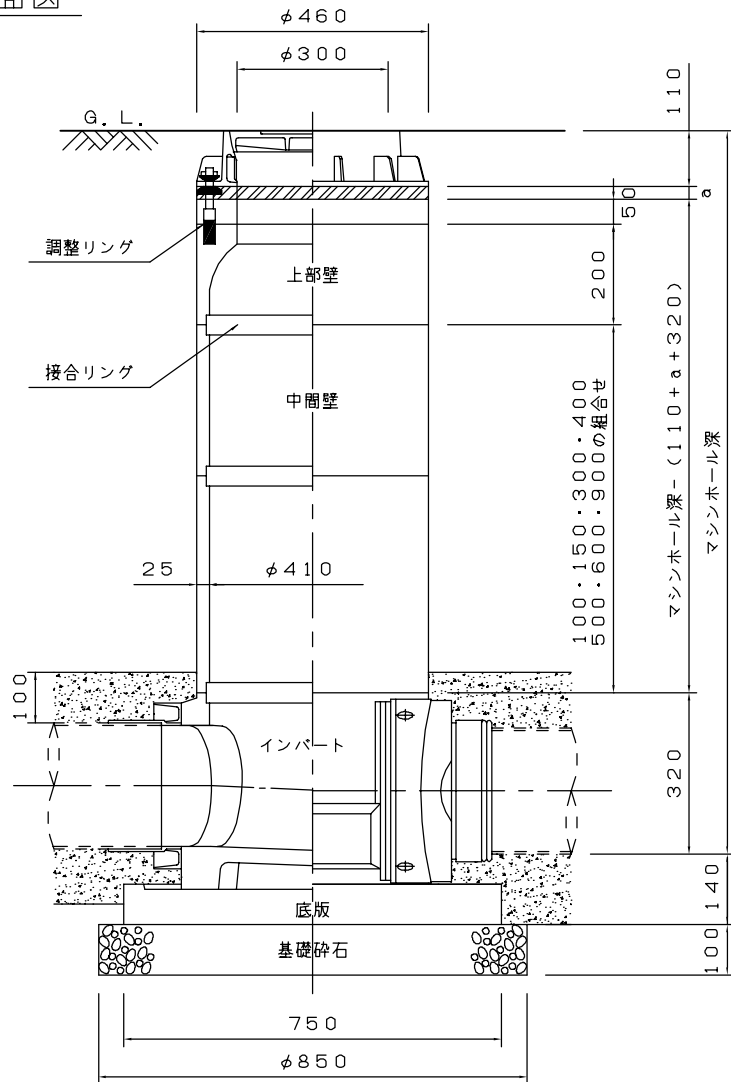
断面図
