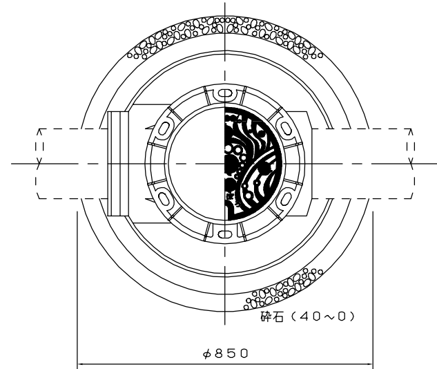
A部詳細
