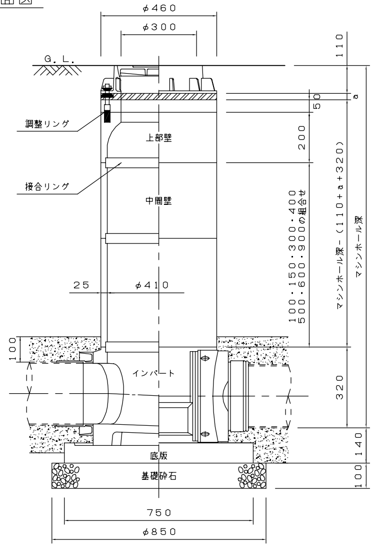
断面図
