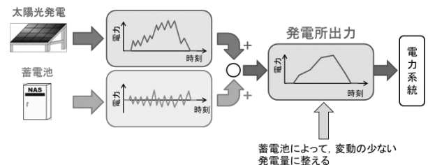
図3 蓄電池による制御
