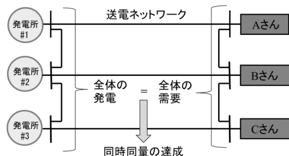
図2 電力系統全体での同時同量
