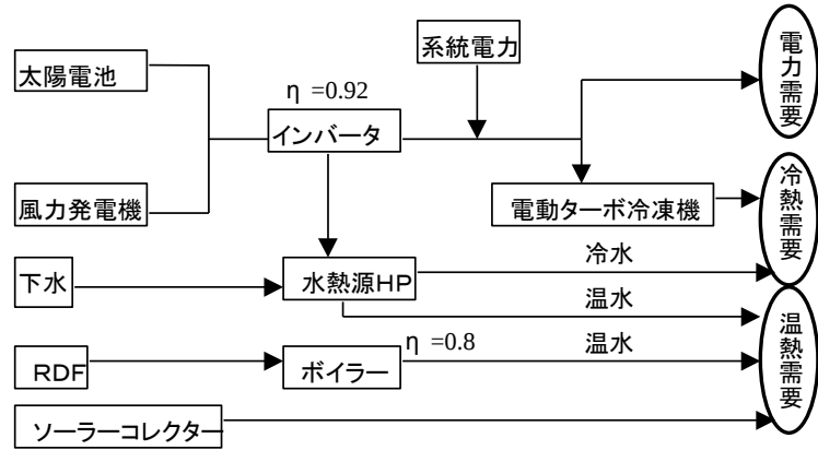
図1.1 地産地消型の再生可能エネルギーの利用システム
