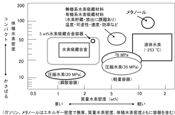
図1 各水素貯蔵技術の水素貯蔵能力
