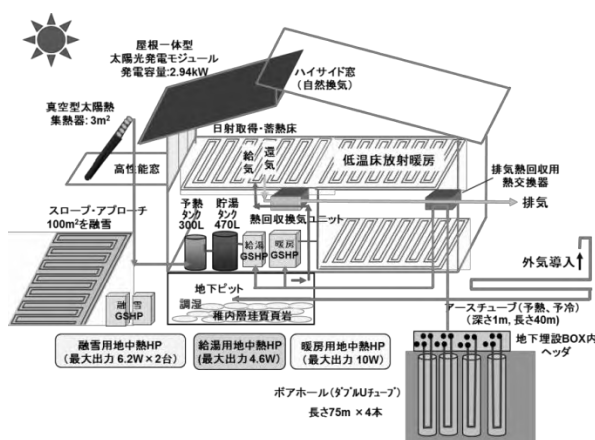
図2.1 環境設備システムの概要
