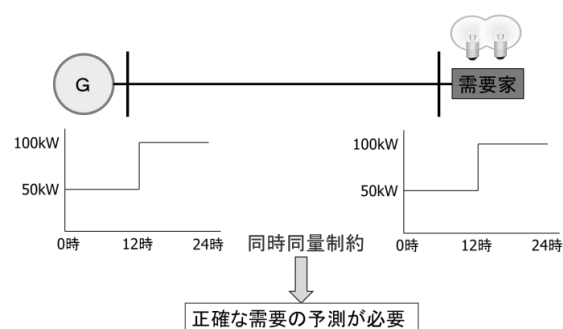
図1 電力の同時同量制約
