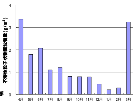
図2 不溶性粒子状物質の沈着量
