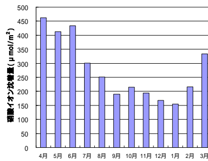
図6 NO 3 - 沈着量の月変化
