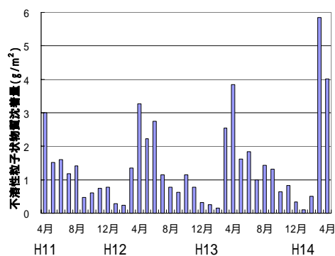
図3 不溶性粒子状物質の沈着量の経年変化
