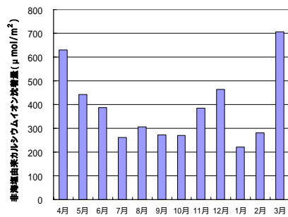
図9 nss-Ca 2+ 沈着量の月変化
