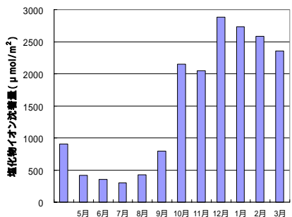
図7 Cl - 沈着量の月変化
