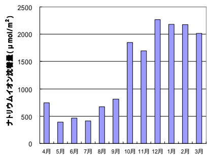
図8 Na + 沈着量の月変化
