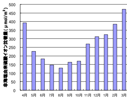
図5 nss-SO 4 2- 沈着量の月変化
