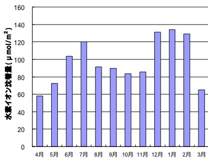
図4 H + 沈着量の月変化
