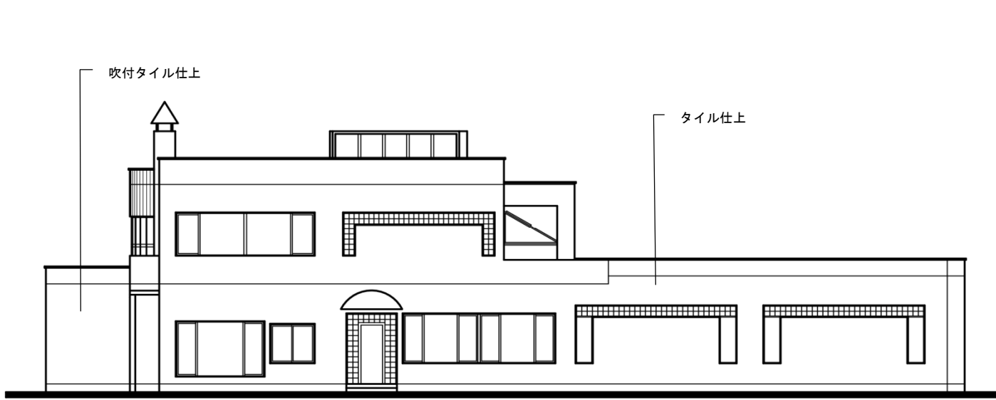
西 立面図
